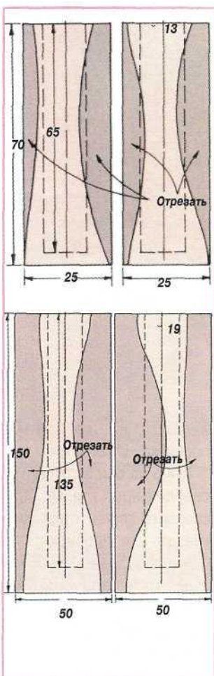
Рис. 2. Контуры обводов корпуса для малой и большой вазы в масштабе 1:1.
