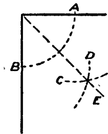
Fig. 323. Halving the Angle.
