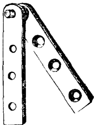
Fig. 235.—Pivot Hinge.
