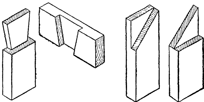
Fig. 33.—Dovetail Halving.
