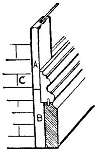
Fig. 119.—Double Skirting Mould.
