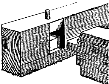
Fig. 152.—Tusk Tenon.
