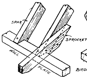
Fig. 354.—Birdsmouth Joint.
