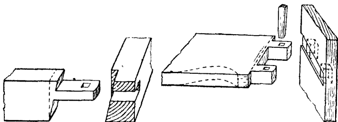
Fig. 154.—Another Type of Tusk Tenon.
