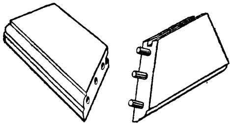
Fig. 202.—Dowelling a Mitred Frame.
