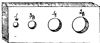
Fig. 190.—Steel Dowel Plate.
