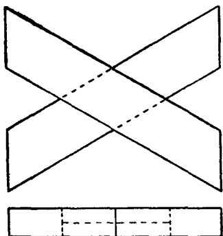
Fig. 51.—Oblique Cross Halving Joint.
