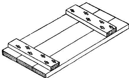
Fig. 367.—Battening.
