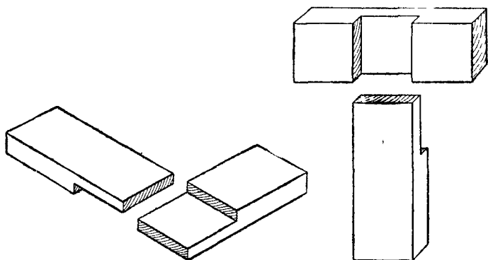
Fig. 29.—Halved Corner Joint. Fig. 30.—Halved T Joint.
