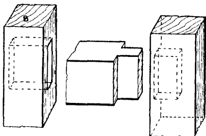
Fig. 128.—Stub Tenon.
