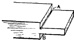
Fig. 145.—Example of Faulty Tenon.
