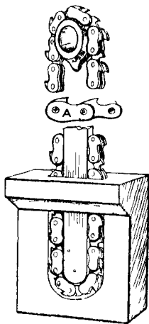
Fig. 139. Sprocket Wheel.
