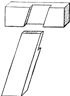
Fig. 32.—Oblique Halving.
