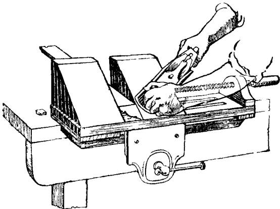
Fig. 326. —The Screw Mitre Trap.
