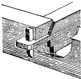
Fig. 153.—Wedged Tusk Tenon.
